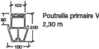
Poutrelle primaire V 1,15 m, 1,50 m, 1,70 m, 3,50 m
