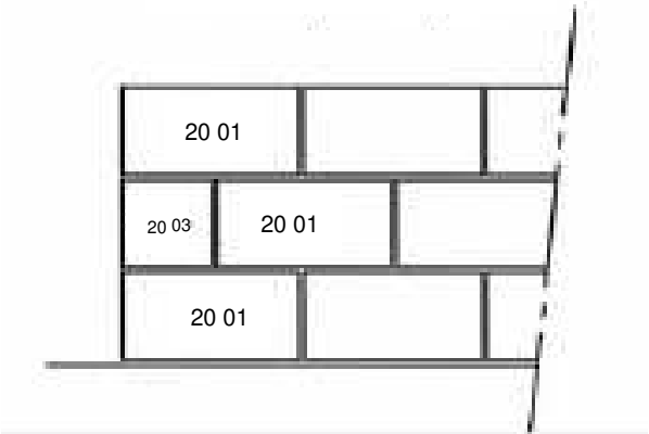
Mur multiple de 0,20 m
