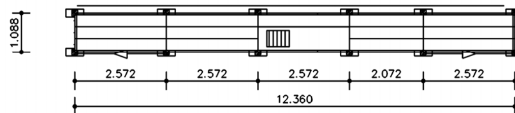
Vue en plan PHASE 3
