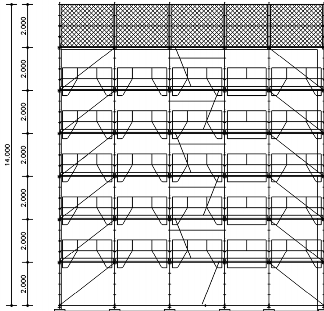
Élévation PHASE 3
