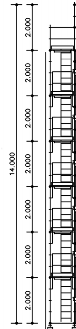
Coupe PHASE 3
